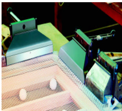
Pneumatische Spanntechnik
